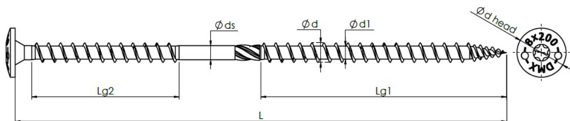
Rysunek 3: Wkręt, typ WKT
