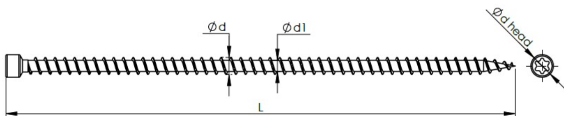
Rysunek 5: Wkręt, typ CPW
